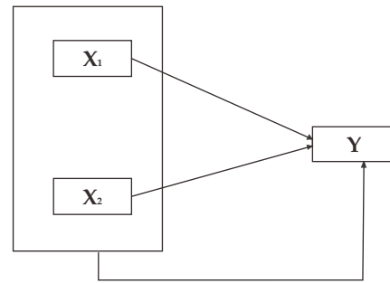
Gambar 3.1. Konstelasi Masalah
